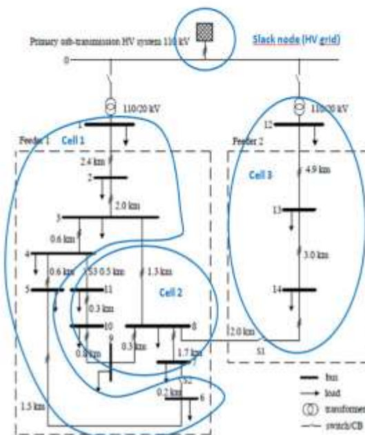
Fig. 1. Test grid (CIGRE MV)
